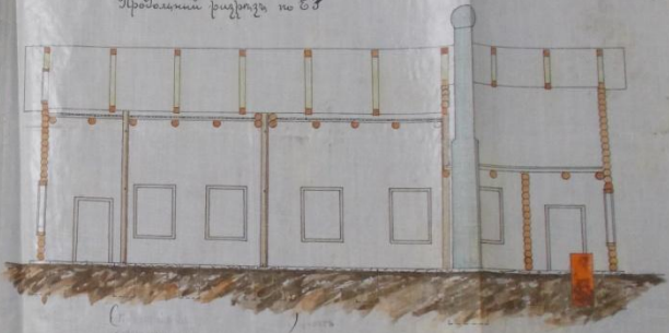
Продольный разрез по ЕФ
