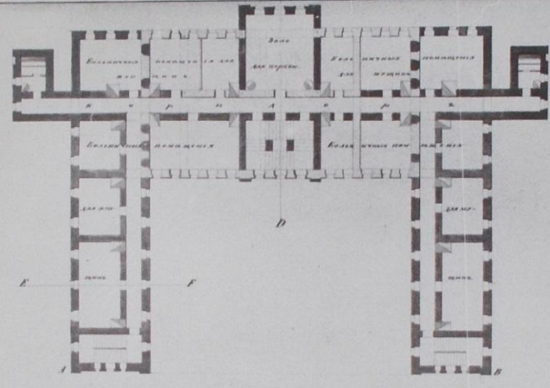
ПЛАНЪ ТРЕТЬЕГО ЭТАЖА, ДОМА.
